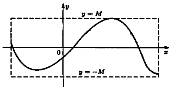
Рис. 1.6. График ограниченной функции.
