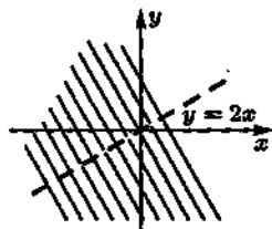
Рис. 3.5. Область определения функции z = (x+y)/(2x-y) .
