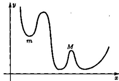
Рис. 2.14. Точки экстремума.
