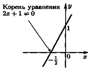
Рис. 1.4. График функции y = 2x + 1 .
