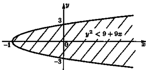
Рис. 3.7. Область определения функции z = \ln(9 + 9x - y^2) .
