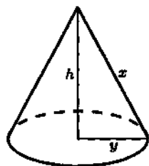
Рис. 3.2. Круговой конус.
