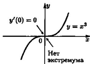
Рис. 2.15. Кубическая парабола.
