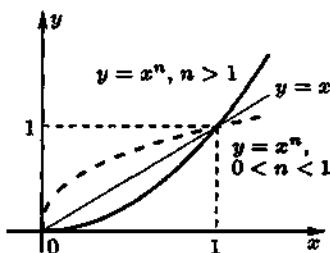
Рис. 1.11а. График функции y = x^n, n > 0 .
