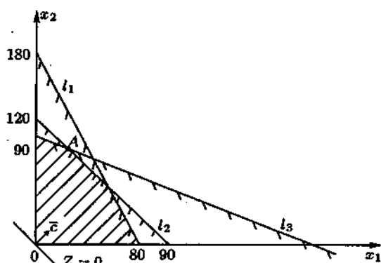
Рис. 9.7. Графическое решение задачи.
