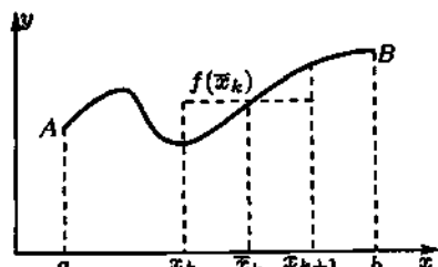
Рис. 5.1. Криволинейная трапеция.
