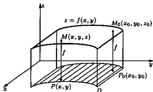
Рис. 3.1. Изображение функции двух переменных в трехмерном пространстве.
